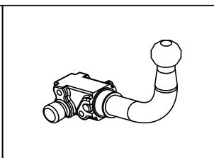
KULA TYP A Kula wypinana poziomo za pomocą dźwigni
