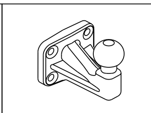
KULA TYP K Płytką z kulą przykręcana za pomocą czterech śrub M12
