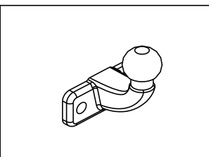
KULA TYP P Płytką z kulą przykręcana za pomocą dwóch śrub M16
